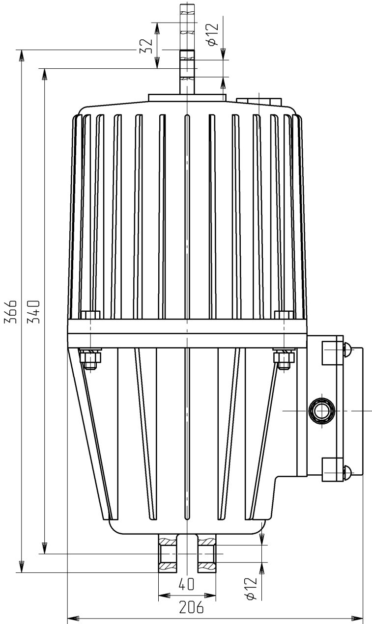
Рис. 1. Габаритные и присоединительные размеры ТЭ-30
