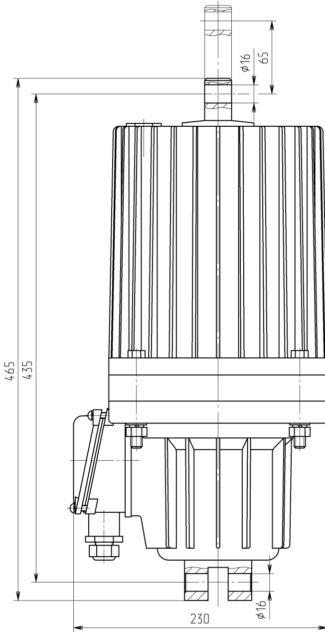
Рис. 1. Габаритные и присоединительные размеры ТЭ-80
